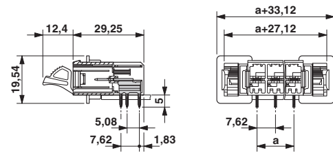
外形寸法
