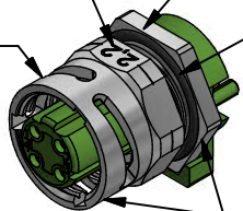
Bayonet nut M12/ Bajonettmutter M12
