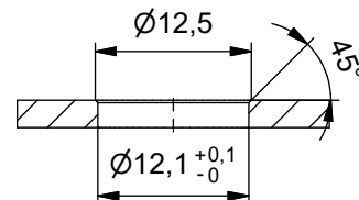
Recommended panel cut-out/ empfohlener Montageausschnitt:
