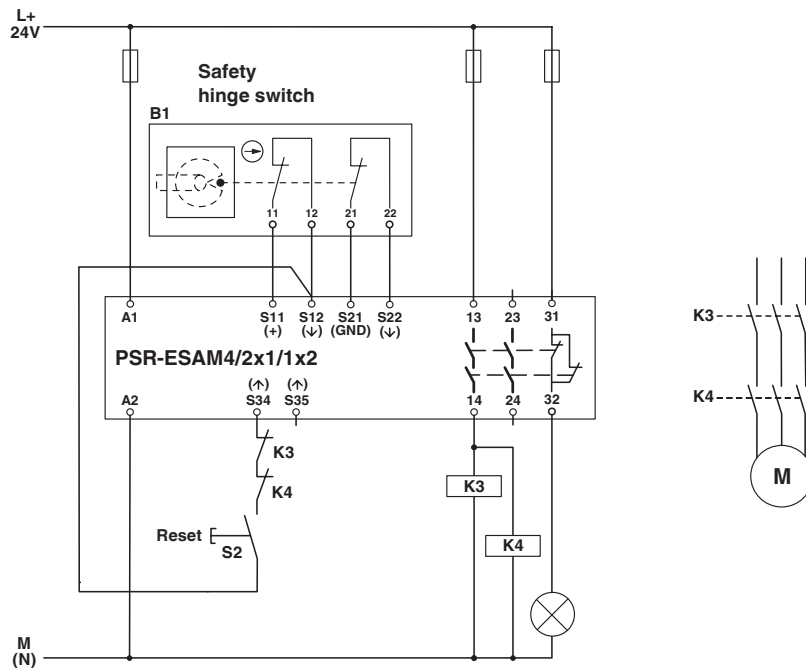
Schaltplan
