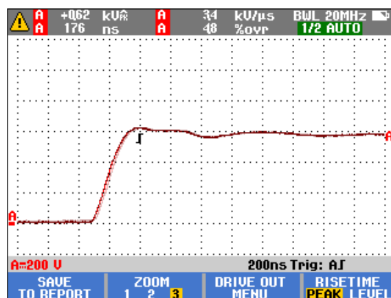
Modulation de la tension avec zoom
