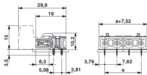
外形寸法
