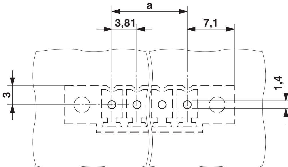
Bohrplan/Lötpadgeometrie
