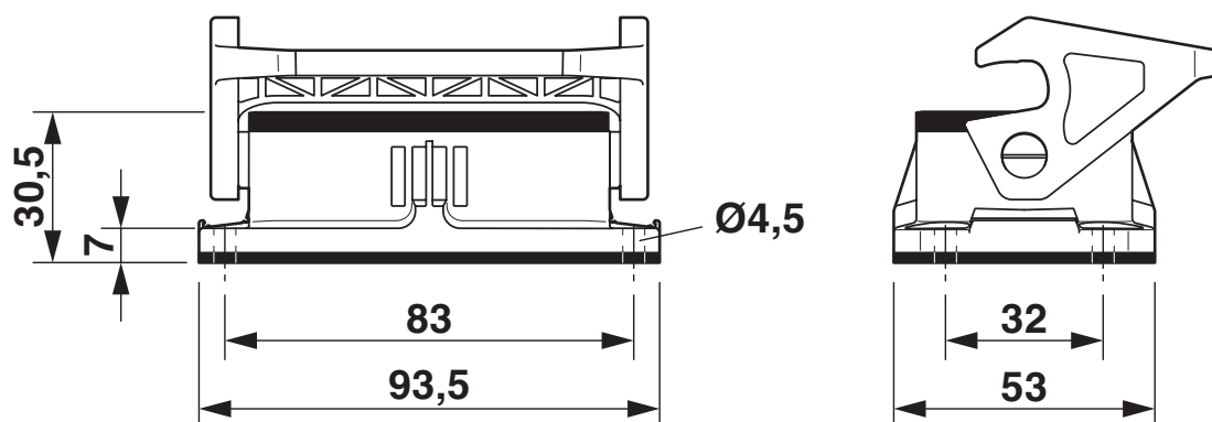
Maßzeichnung
