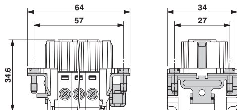
外形寸法
