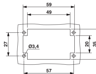
ハウジングを使用しない場合の取付け断面
