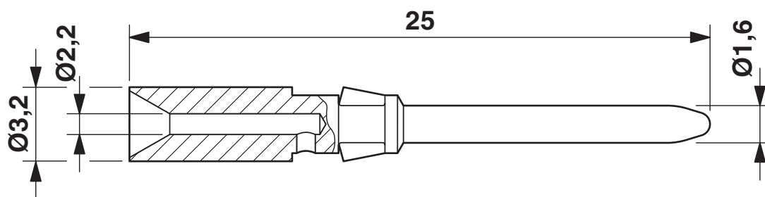
尺寸图
