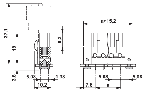
外形寸法
