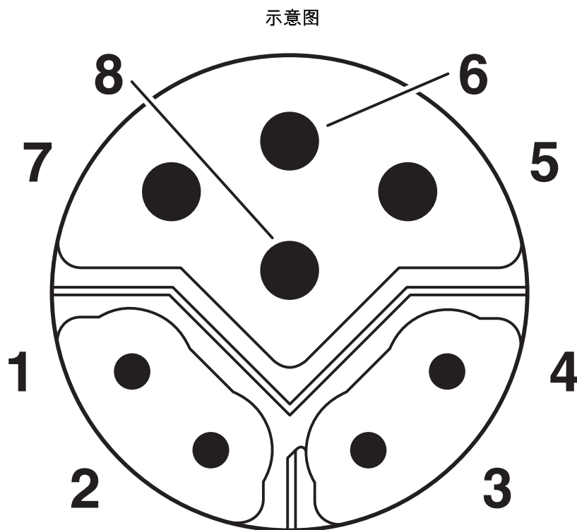
M12混合针式连接器引脚分配，8芯，Y编码，插头侧视图
