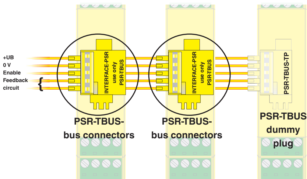
接线图
