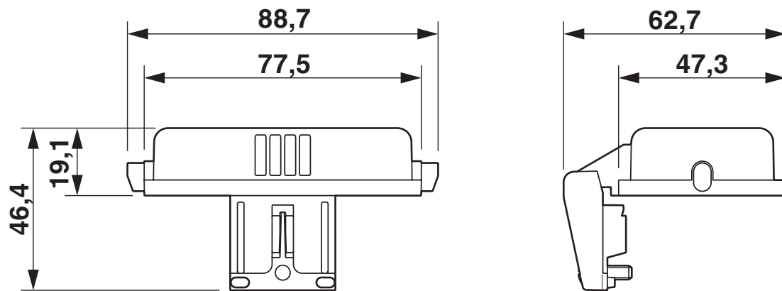
尺寸图
