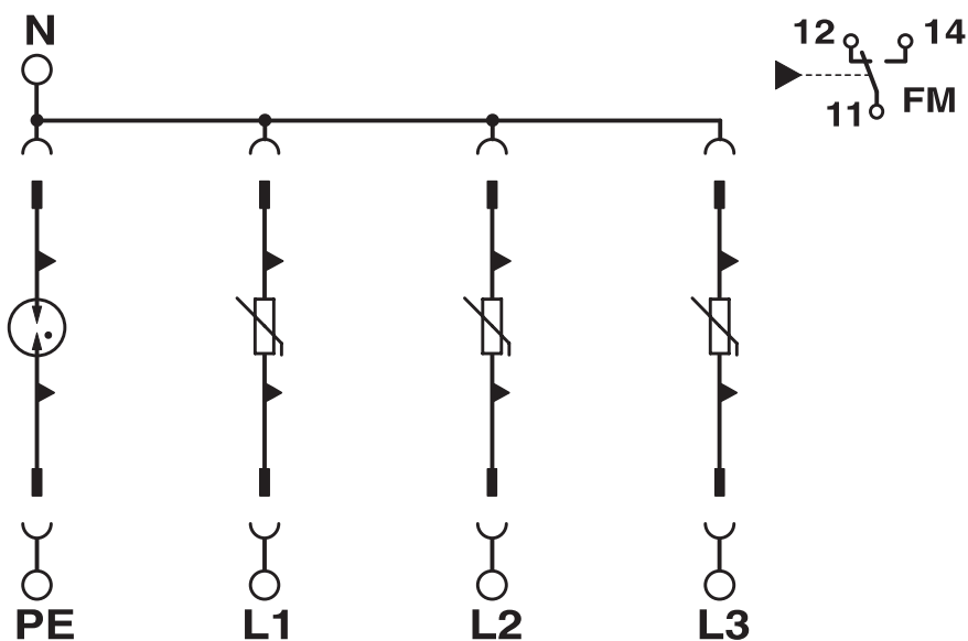
电路图
