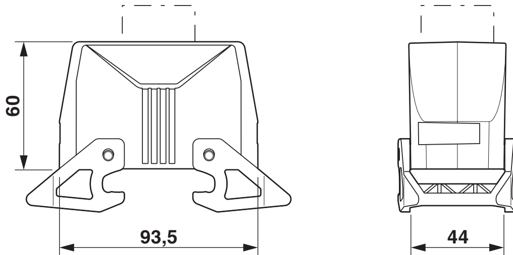
尺寸图
