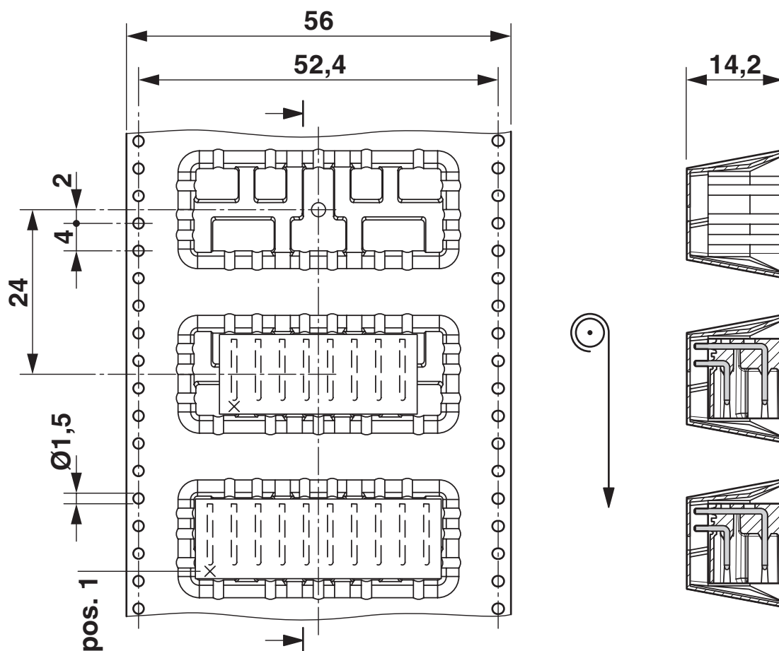
尺寸图
