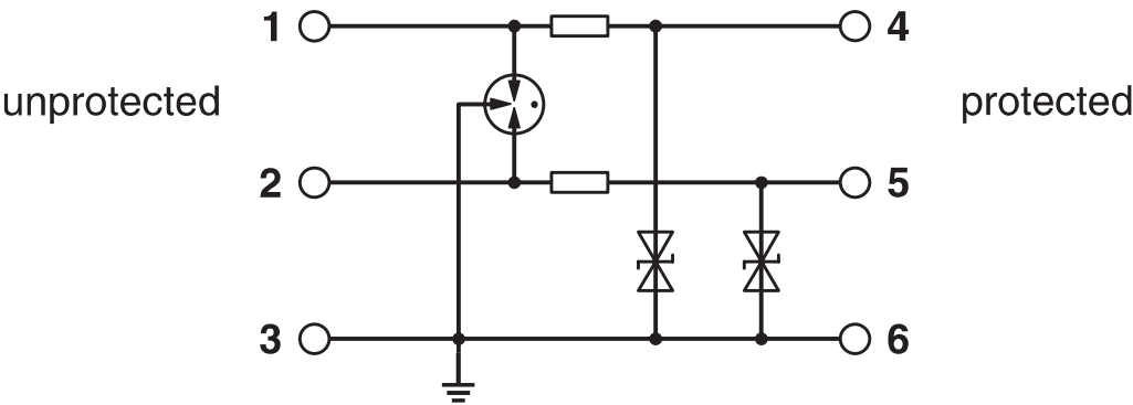
电路图
