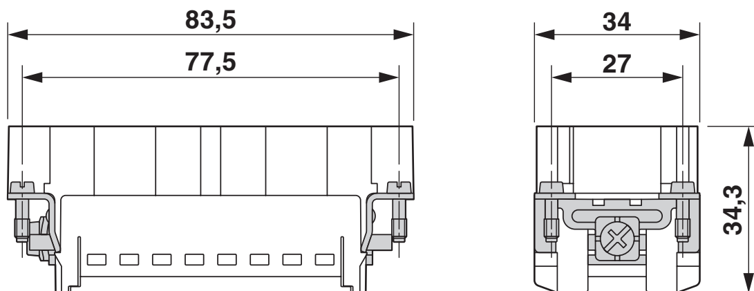
尺寸图
