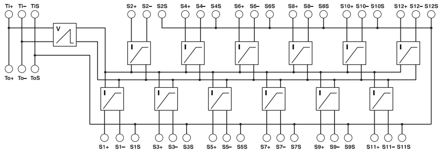
电路图
