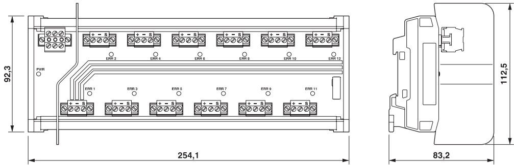
尺寸图
