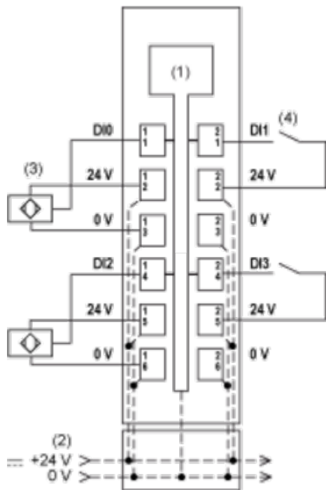
接线图
