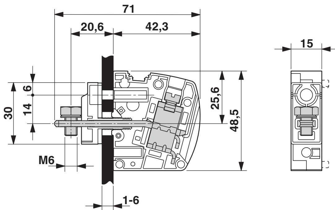
尺寸图
