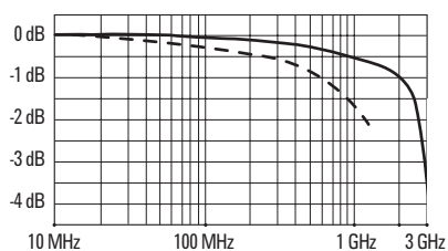
Perte d'insertion
