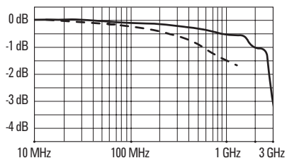
Perte d'insertion
