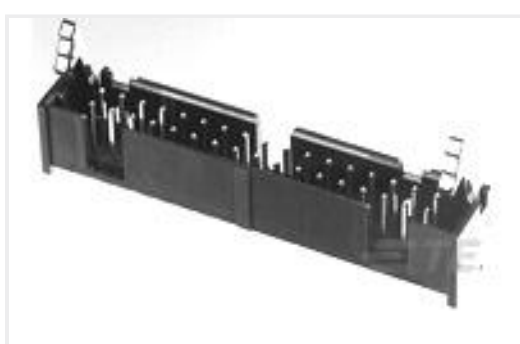
TE Part #2-1761606-3 IDC LOW PRO HDR 10P VERT LAT BLUE
