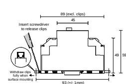
MOUNTING DETAILS INSTRUCTIONS DE MONTAGE MONTAGEAUFÜHRUNGEN
