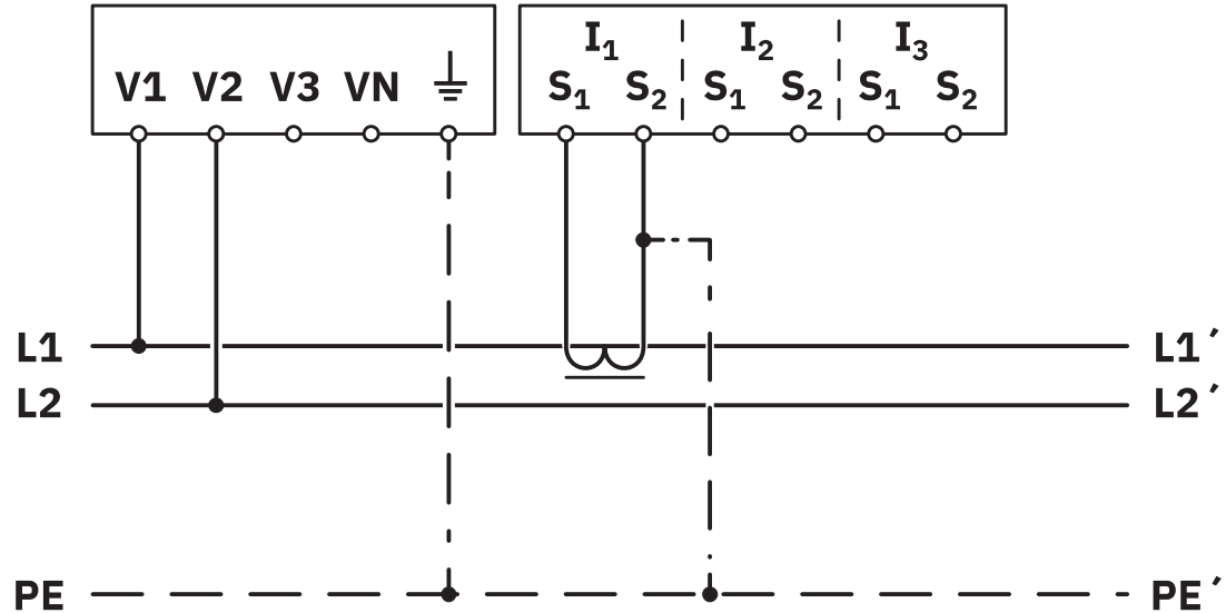
接线图
