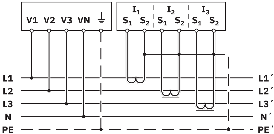
网络类型：3PH-4W-3CT
