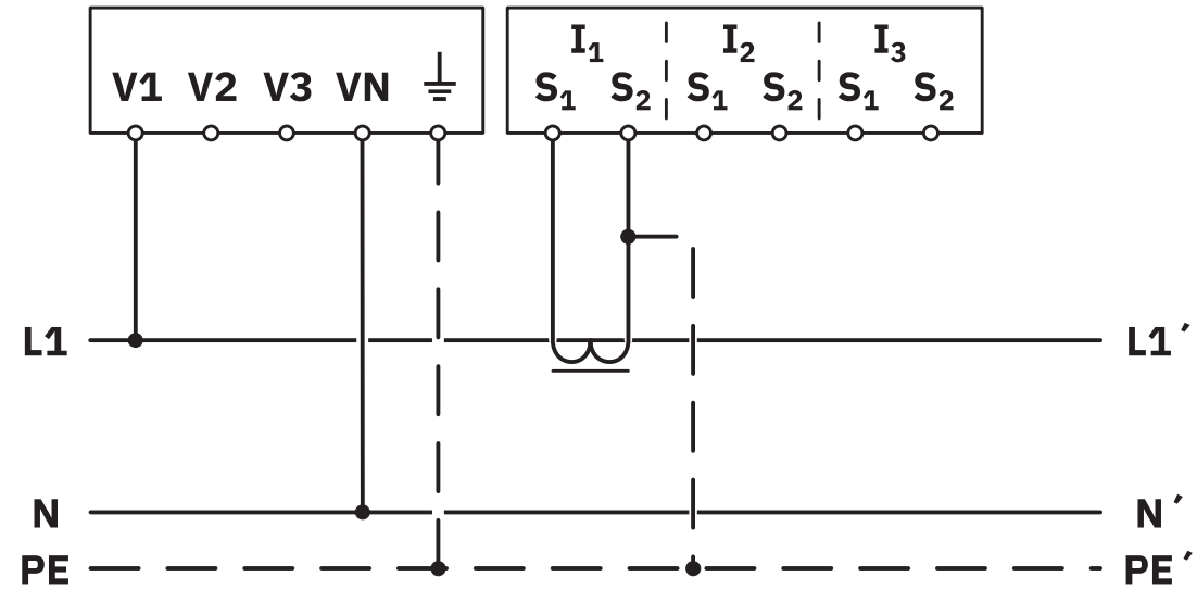
网络类型：1PH-2W-1CT
