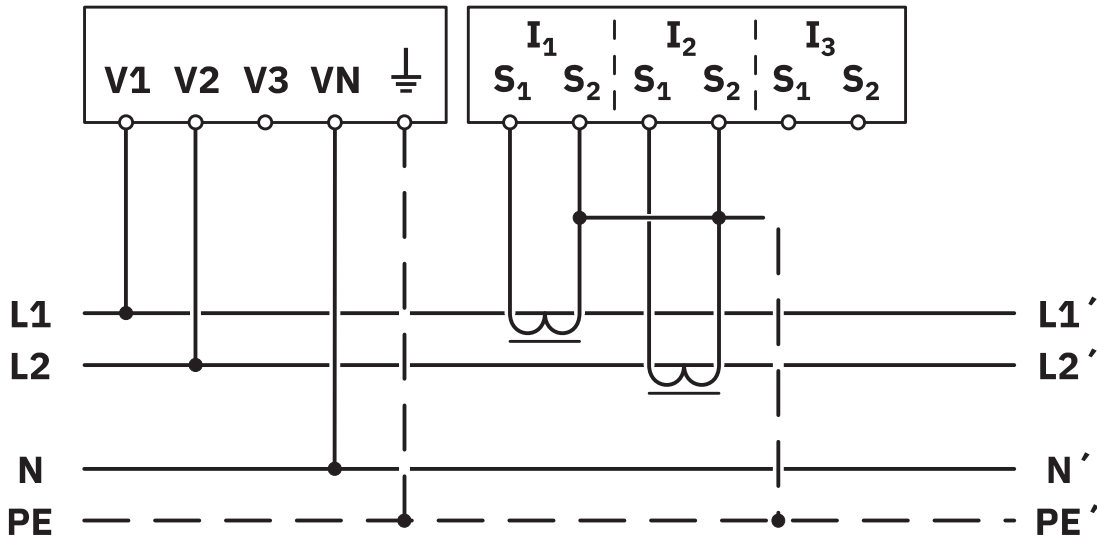
接线图
