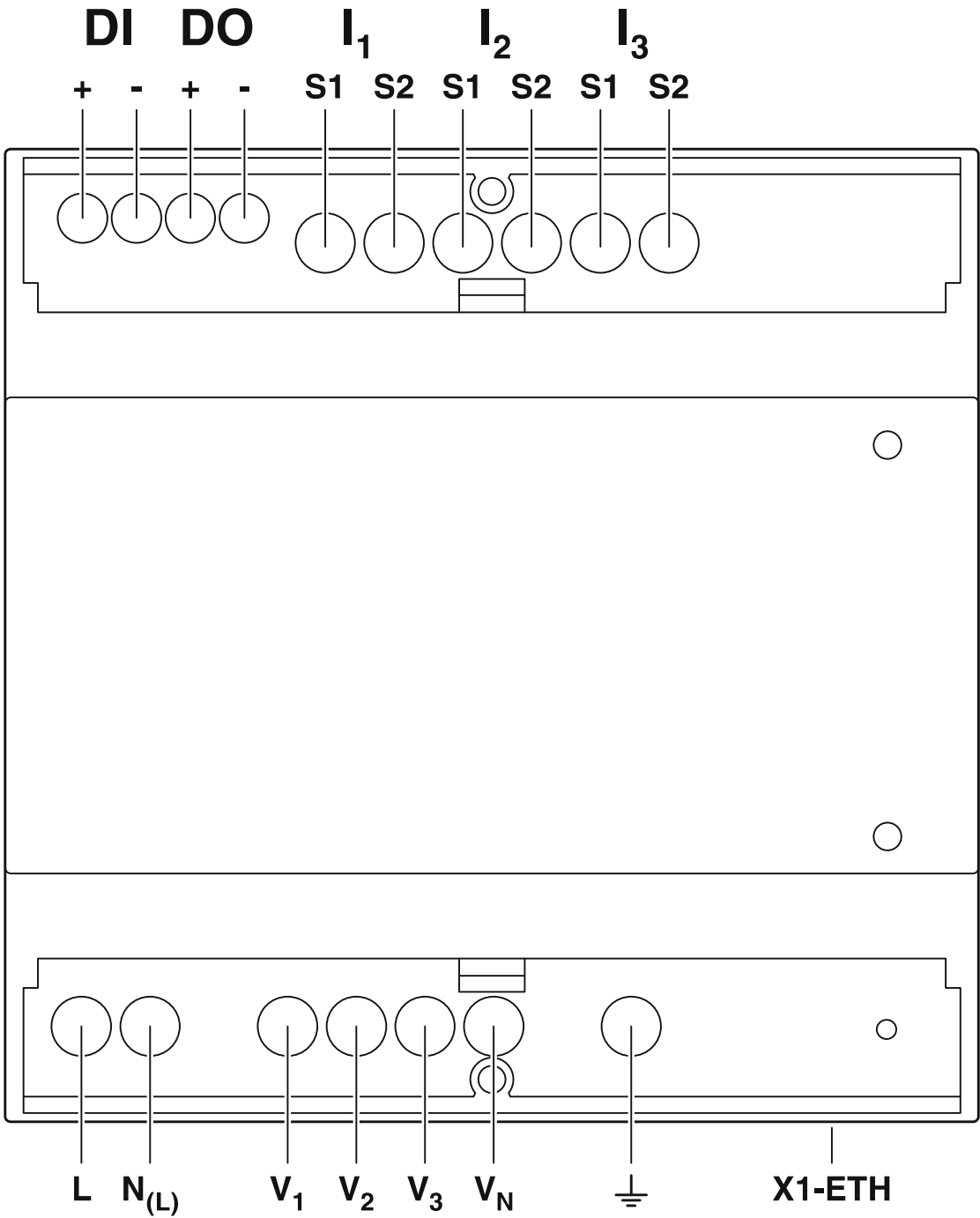
接线图
