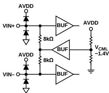
Figure 14. Analog Inputs ( V_{CM} \approx 1.4V )
