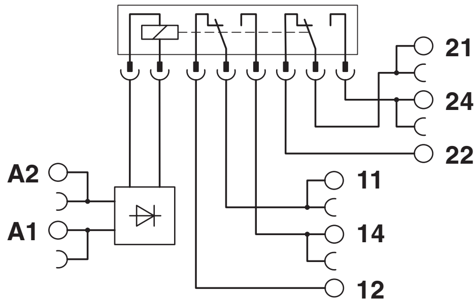
电路图
