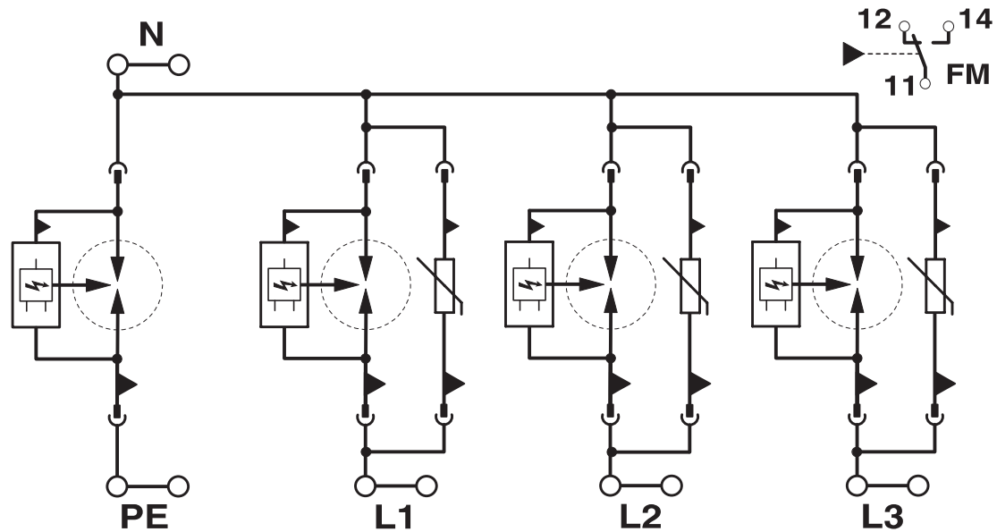
电路图
