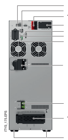
ITYS 6 - 10 kVA - 1/1
