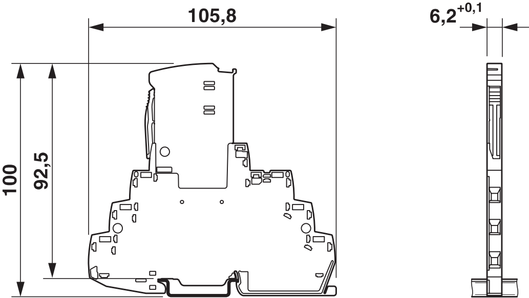
尺寸图
