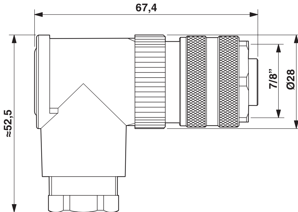
尺寸图
