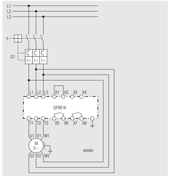
Softstart in a \sqrt{3} -circuit
