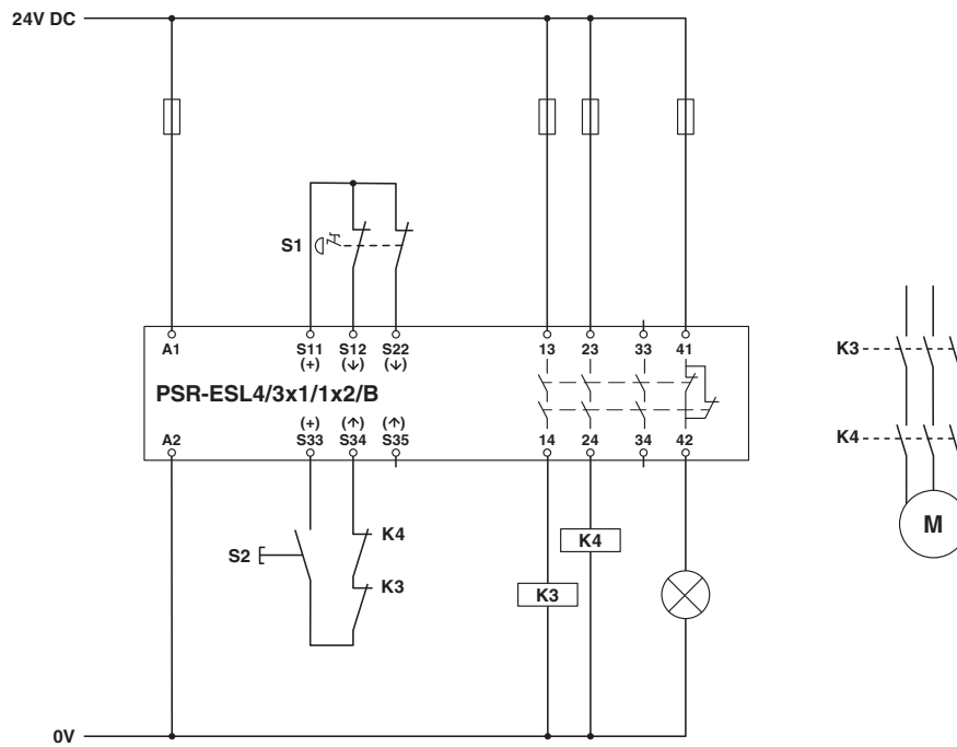
Schaltplan
