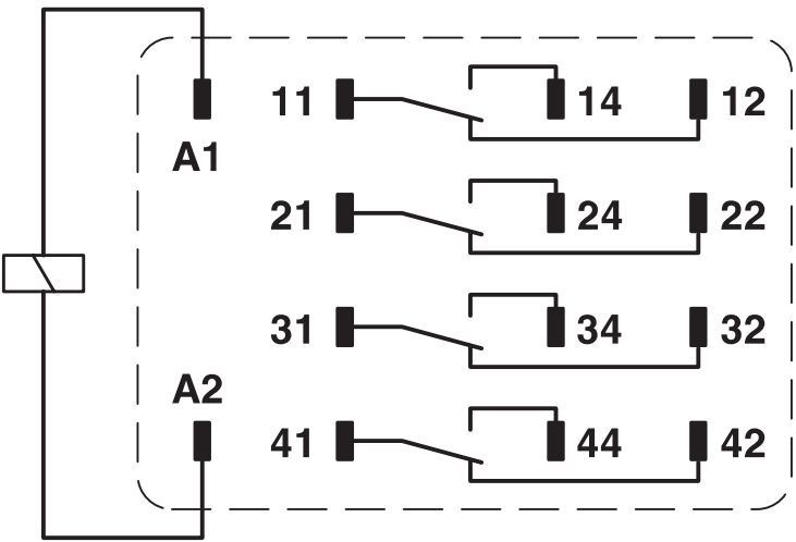
电路图
