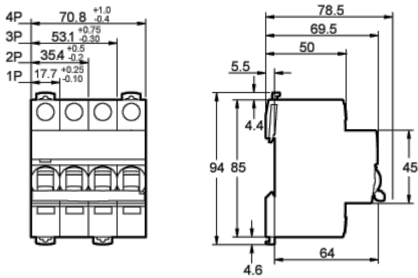
尺寸(mm)
