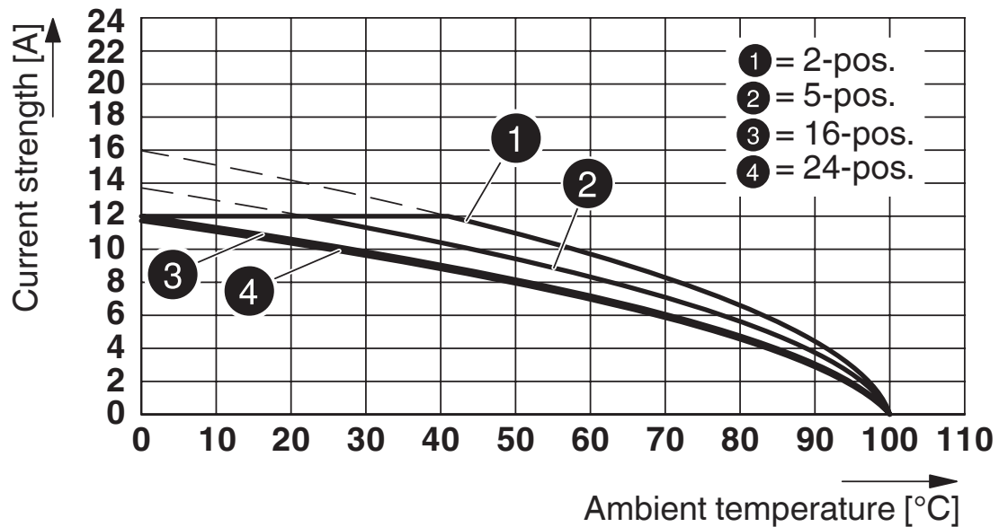
Typ: MVSTB(R/W) 2,5/...-ST mit MSTBV 2,5/...-G
