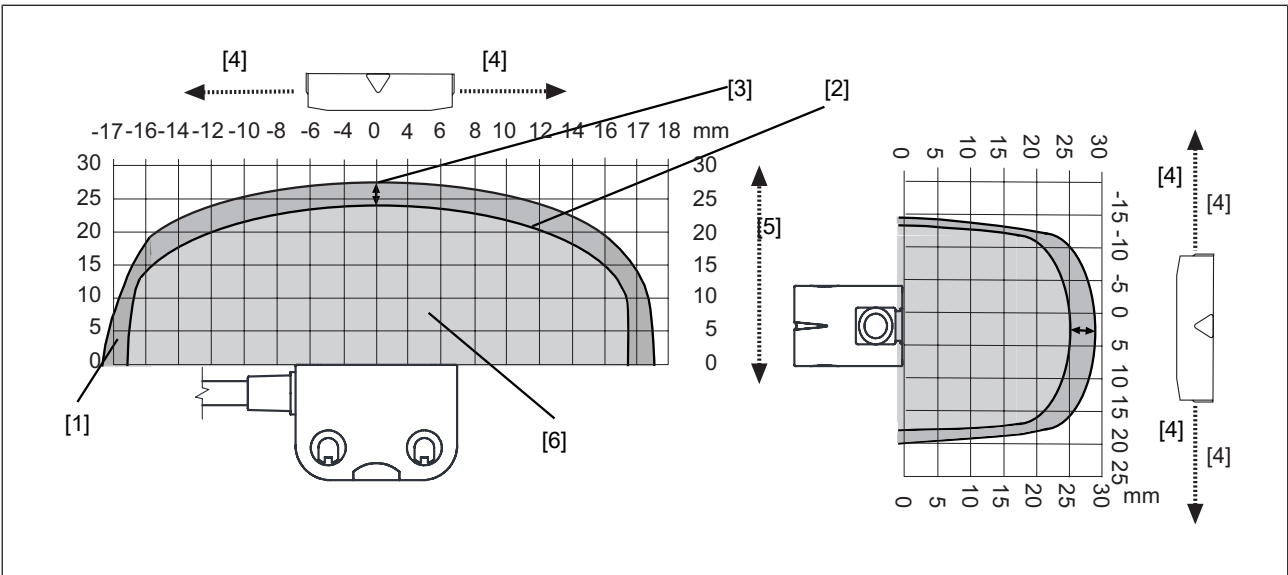
Abb.: Sicherheitsschalter PSEN cs3.1a/b mit Betätiger PSEN cs1.1
