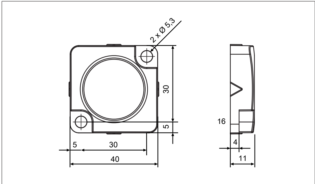
Abb.: Betätiger PSEN cs1.1
