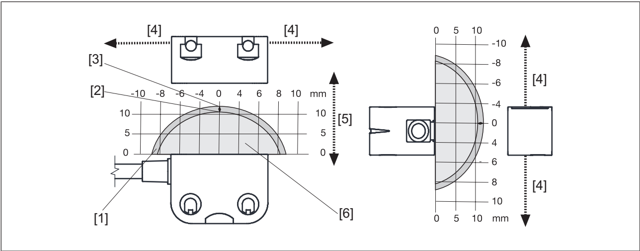
Abb.: Sicherheitsschalter PSEN cs3.1a/b mit Betätiger PSEN cs3.1
