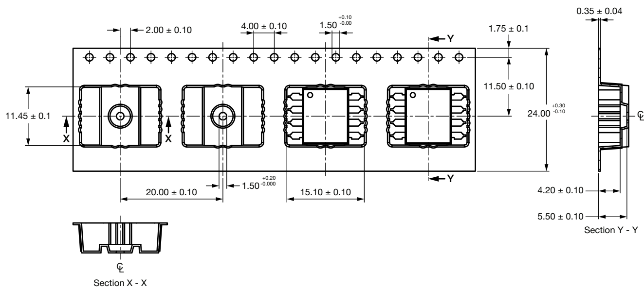
Fig. 20 - Tape Dimensions
