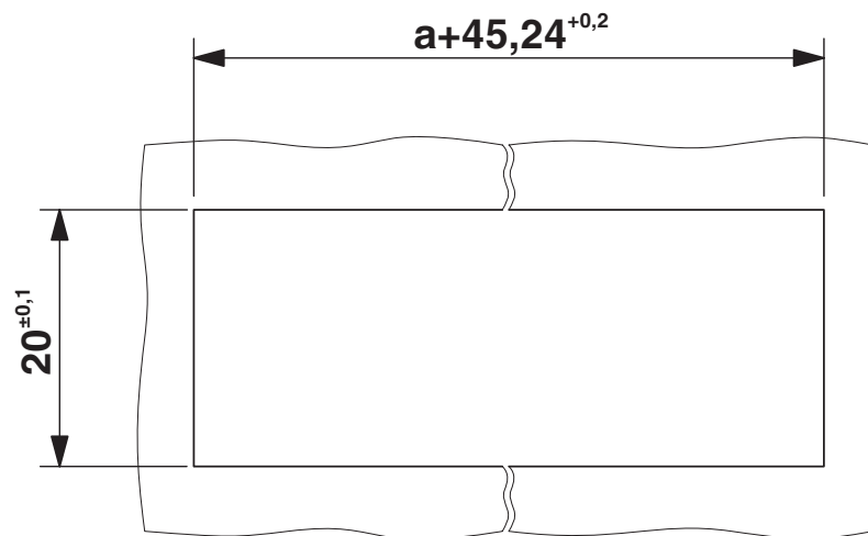
尺寸图
