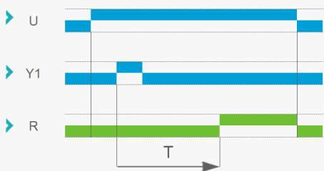
Fonction Ah : Clignotant cycle unique par commande
