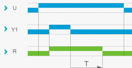
Fonction D : Clignotant à cycle symétrique (départ OFF)
