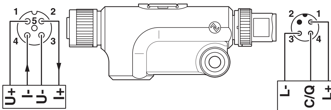
Anschlusszeichnung
