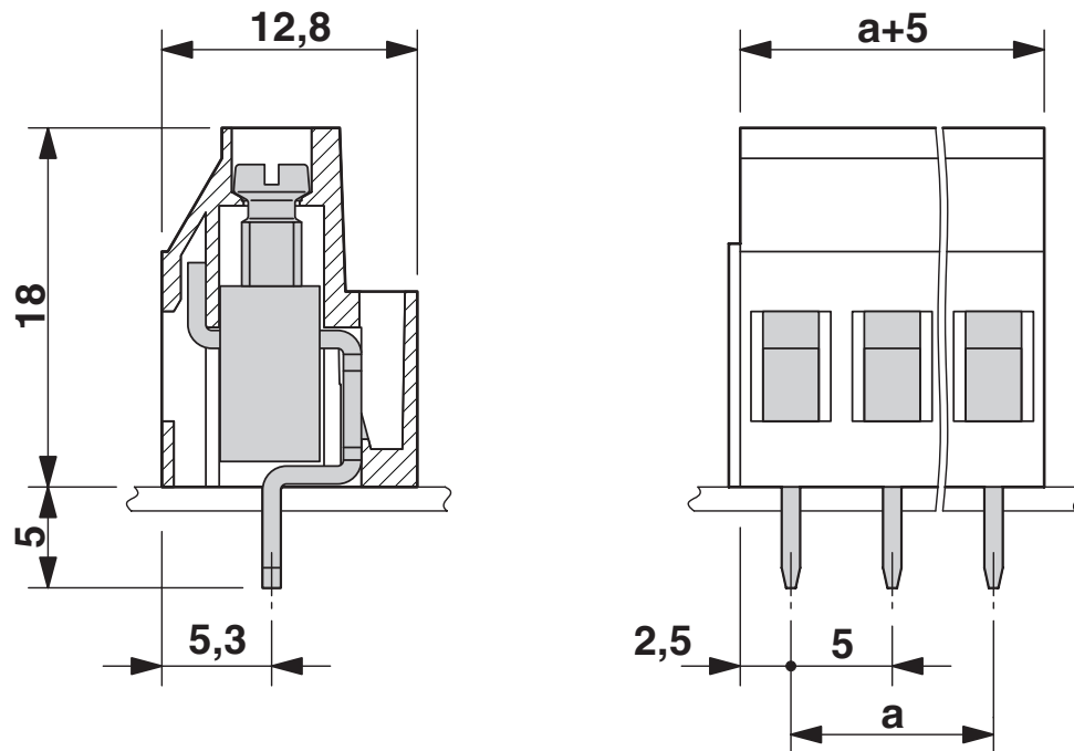
尺寸图
