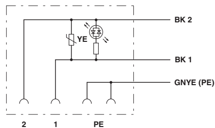
回路図
