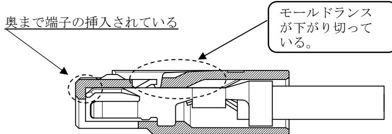
Fig.6-4 正しく装着されている場合
