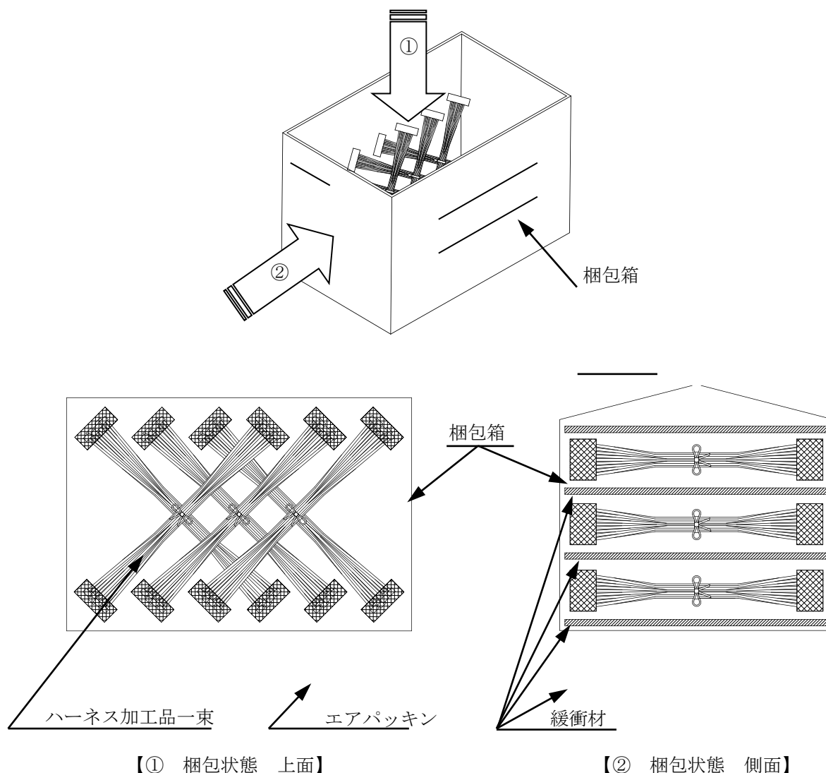
Fig.8-2 梱包状態図
