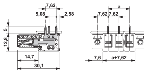
外形寸法
