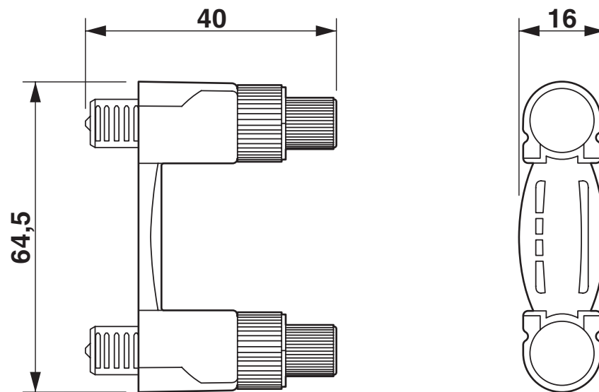
Maßzeichnung
