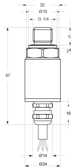
Cable output
