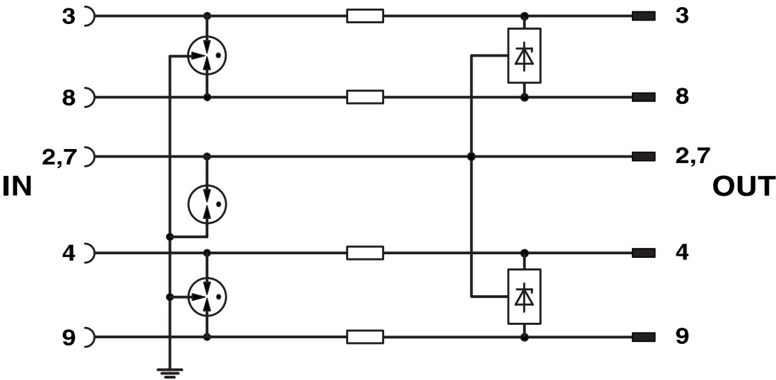
电路图
