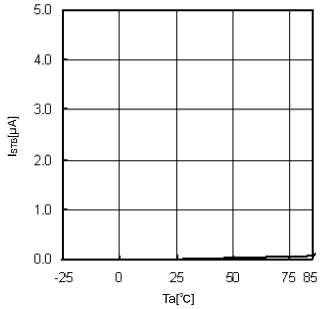
Fig.12 Ta-Istb (VEN=0V)
