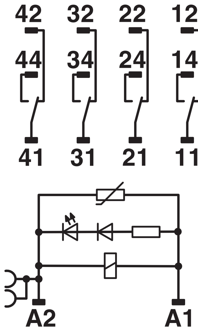
电路图
